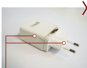
Sinais de ruptura (causados por quedas ou choques físicos)
