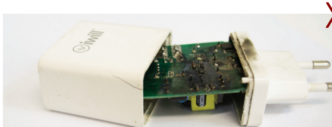
Este carregador foi desmontado e montado novamente de maneira invertida, levando ao curto do sistema
